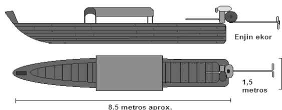
Ilustración 3: Estructura de un perahu
